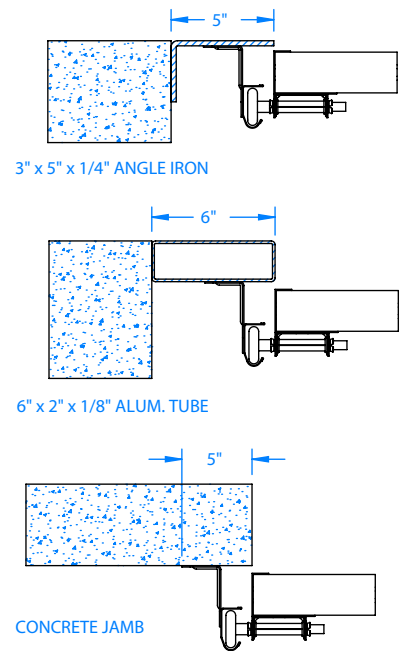
JAMB PLAN DETAIL
